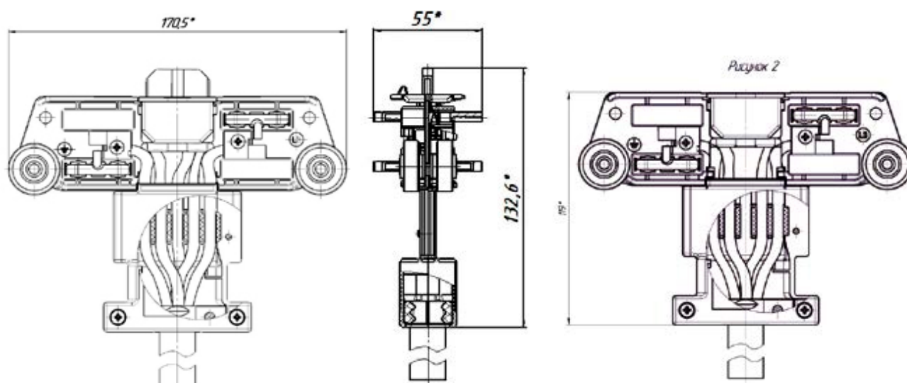
Технические характеристики: токоъемник 21-485-01 троллейного шинопровода
