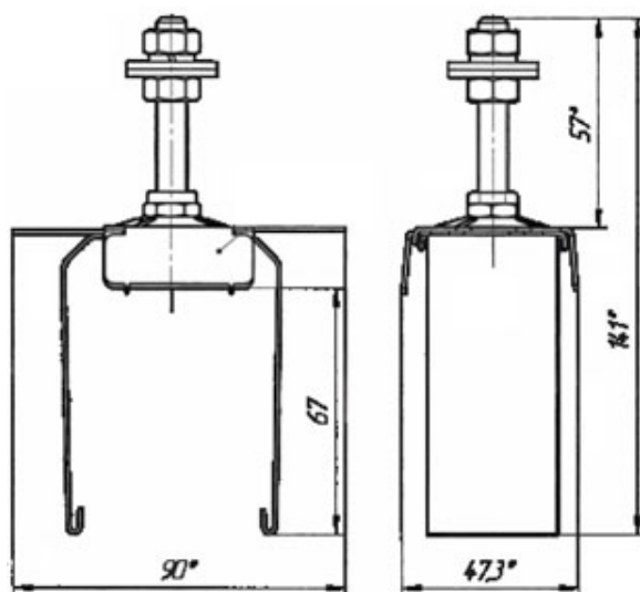
Технические характеристики: подвес жесткий 21-485-04 троллейного шинопровода
